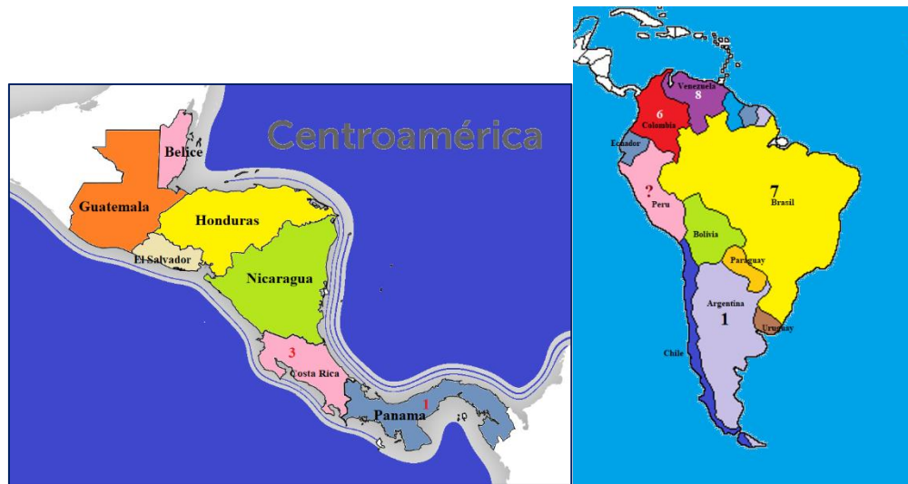
Figura N° 2: Distribución de casos reportados en latino américa de PAM por Naegleria fowleri .
